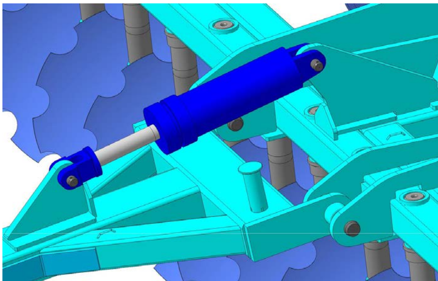
Усиленная сница
