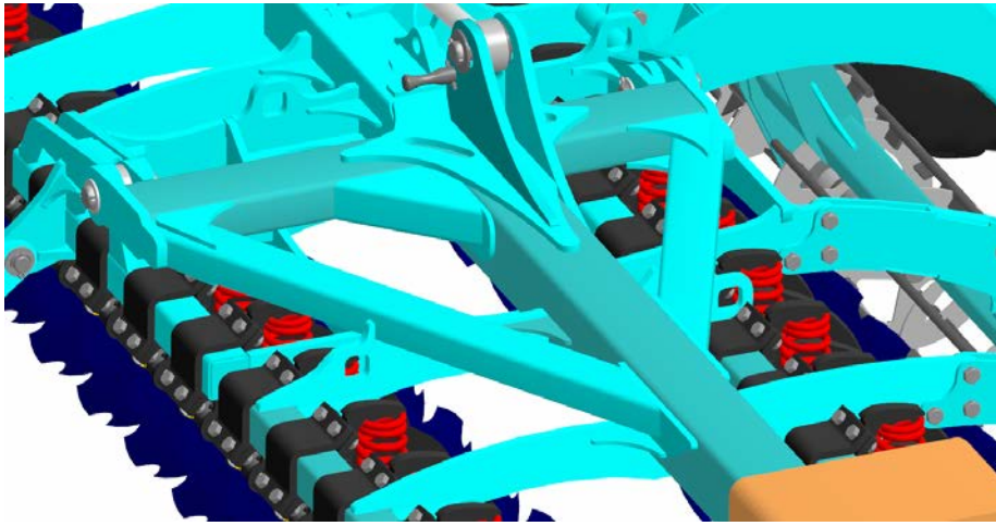
Мощное крепление сноты к раме.
